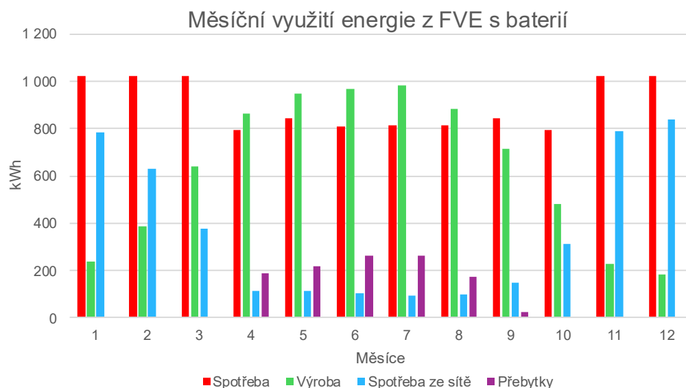
Obr. 32 Měsíční využití energie z FVE s baterií
