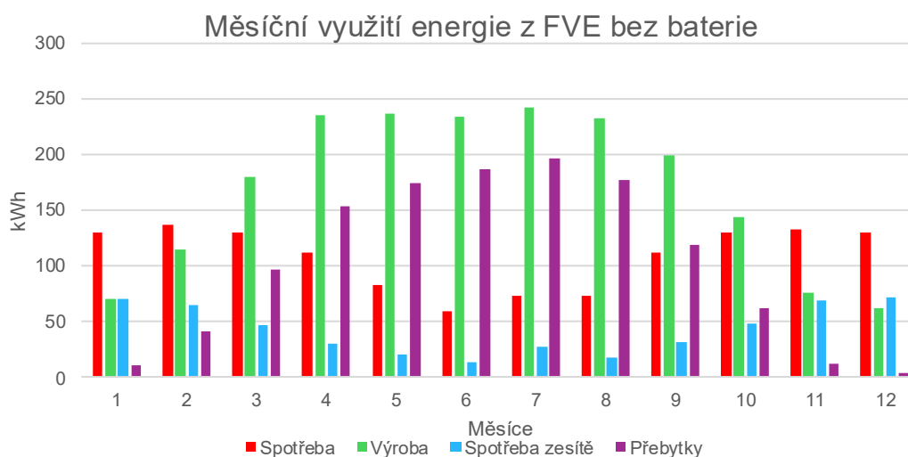
Obr. 34 Měsíční využití energie z FVE bez baterie
