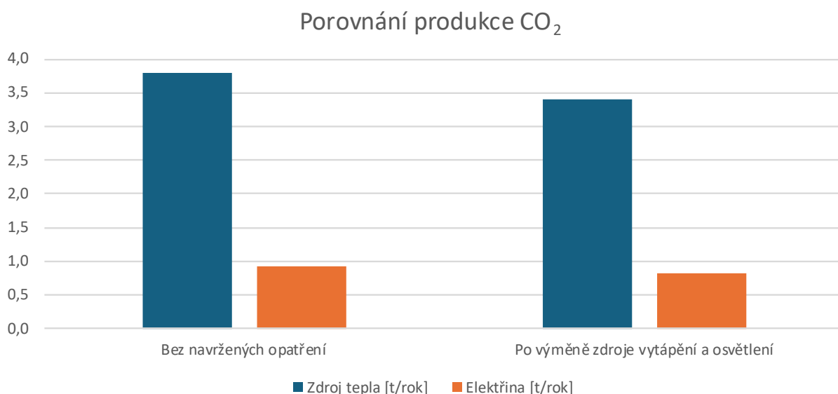
Obr. 30 Uhlíková stopa návrhových opatření
