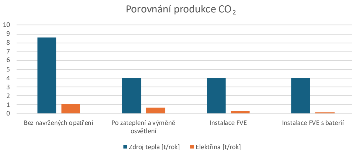
Obr. 36 Uhlíková stopa návrhových opatření
