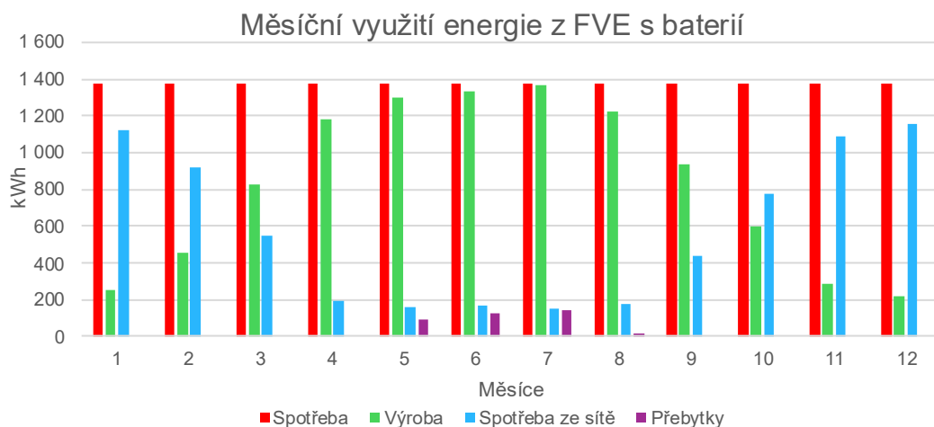
Obr. 38 Měsíční využití energie z FVE s baterií
