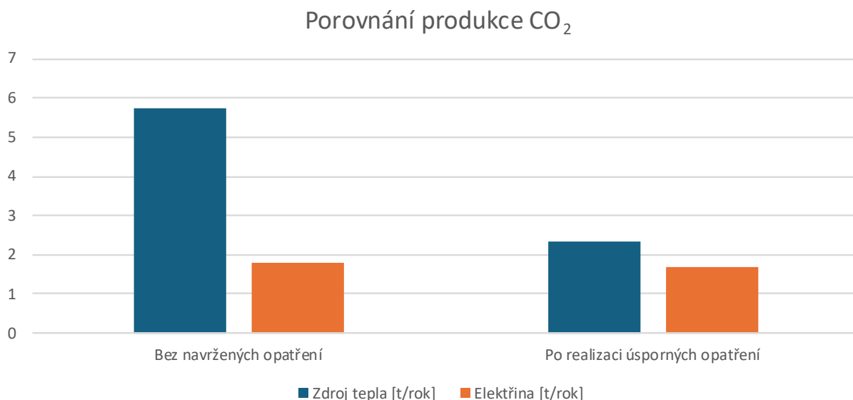
Obr. 29 Uhlíková stopa návrhových opatření
