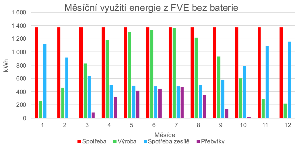
Obr. 37 Měsíční využití energie z FVE bez baterie
