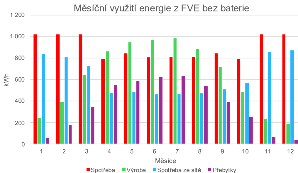
Obr. 31 Měsíční využití energie z FVE bez baterie
