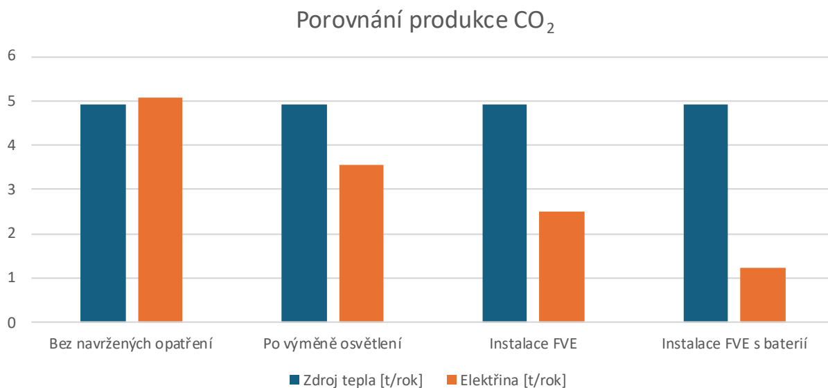
Obr. 33 Uhlíková stopa návrhových opatření
