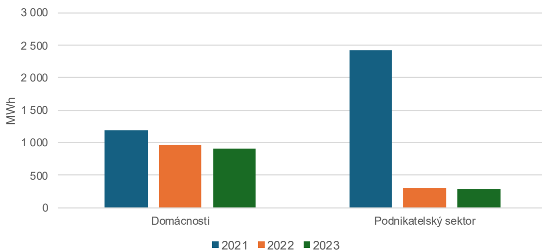
Obr. 10 Spotřeba plynu soukromý sektor
