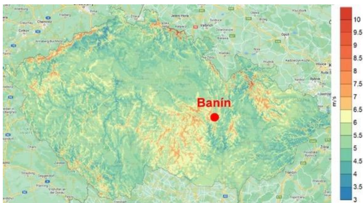
Obr. 15 Přehledová mapa potenciálu větru ve 100 metrech výšky nad povrchem (zdroj: Ústav fyziky atmosféry AV ČR, v. v. i.)
