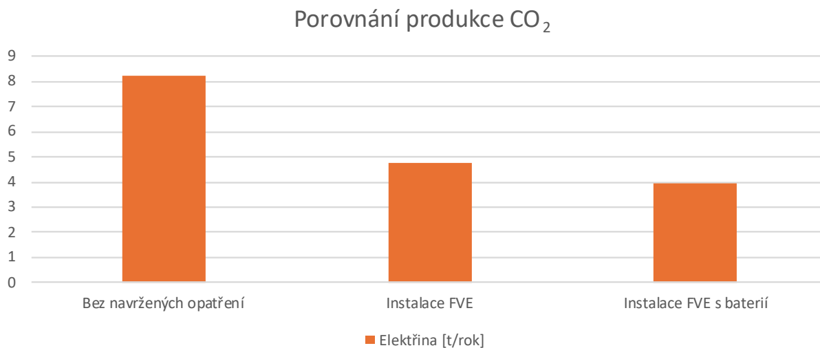
Obr. 39 Uhlíková stopa návrhových opatření
