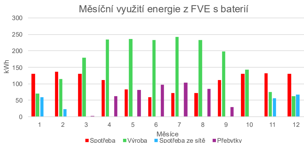
Obr. 35 Měsíční využití energie z FVE s baterií
